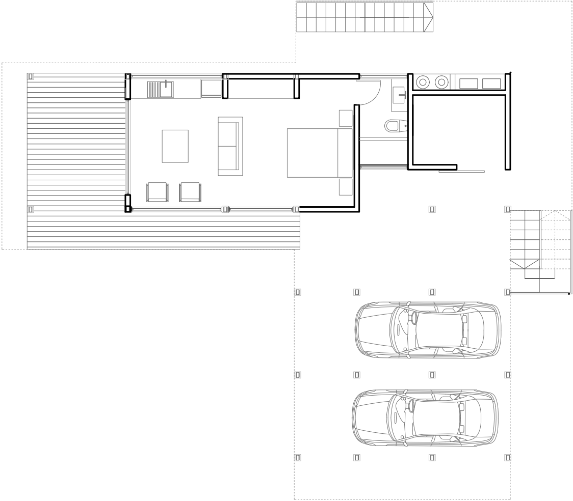
Planta Arquitectura N° -1 Casa PPL 2 Esc 1:50
